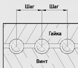
Рис 4.18 Преднатяг заданный диам. шарика
