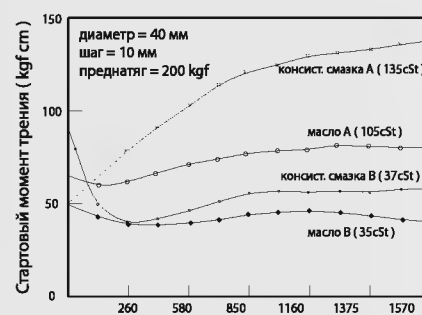
Рис 4.31 Влияние вязкости смазки на момент трения
