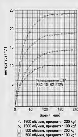
Рис 4.29 Связь рабочей скорости, преднатяга и рост температуры
