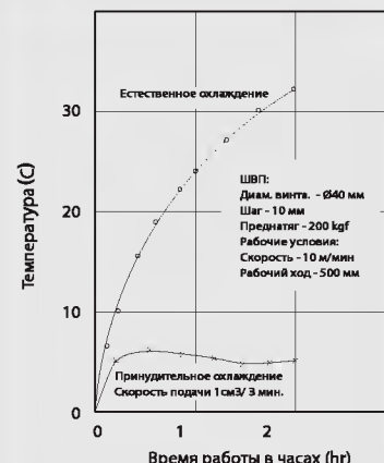
Рис 4.32 Повышение температуры ШВП с охлаждением и без него
