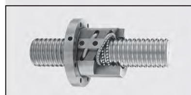
Рис 3.1 Наружный тип рециркуляции шариков с возвратной трубкой
