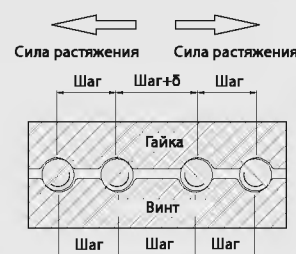
Рис 4.19 Преднатяг типа "Offset"
