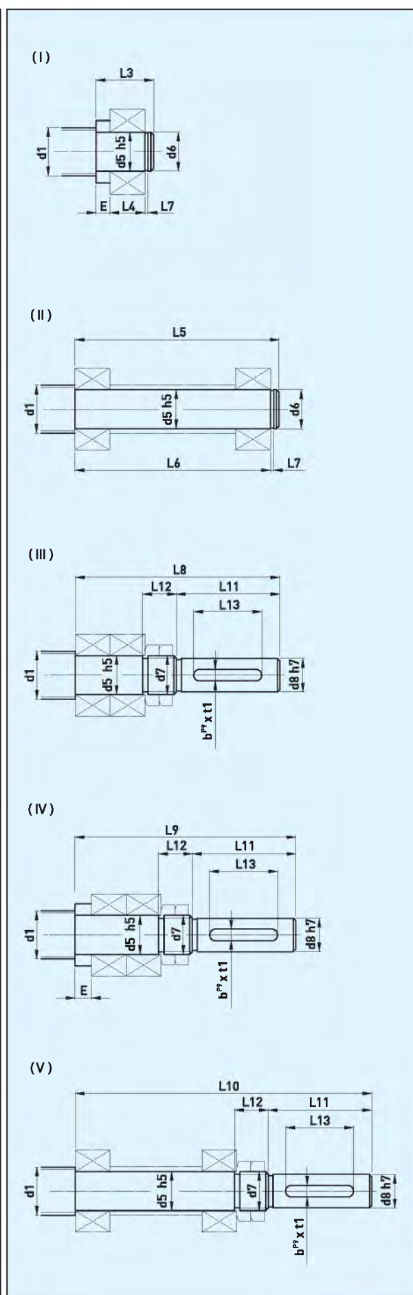
Рис 3.7 Конфигурации концов винта
