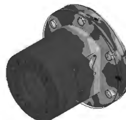
Термический анализ гайки с охлаждением
