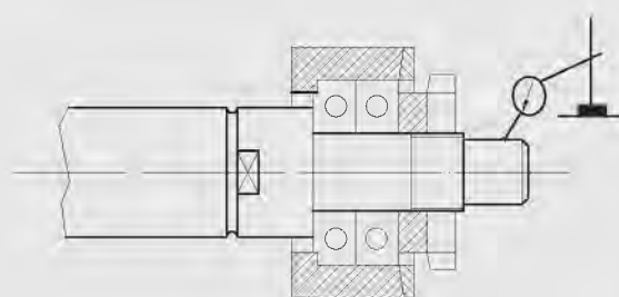
Рис А-3 Замеры осевого отклонения шейки винта
