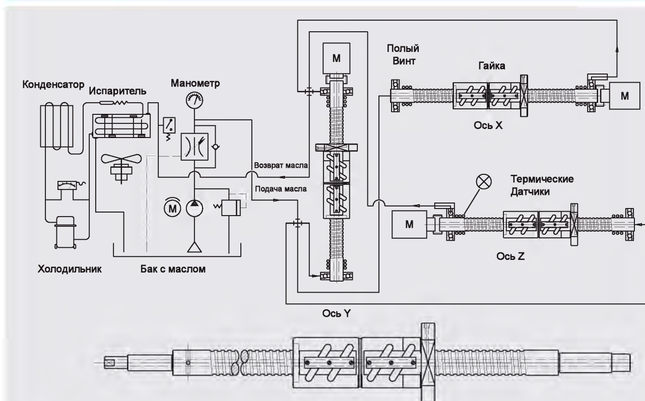
Рис 4.33 Пример системы высокого класса точности с применением полого винта для охлаждающей жидкости
