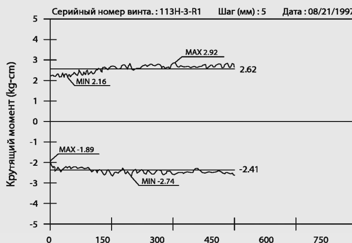
Диаг. 2.5 HIWIN проверка преднатяга.
