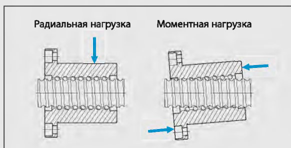
Рис 4.2(а) Дисбаланс в системе вызванный несоосностью её элементов: подшипниковых опор и гайки ШВП проблемы с корпусом гайки и т.д.
